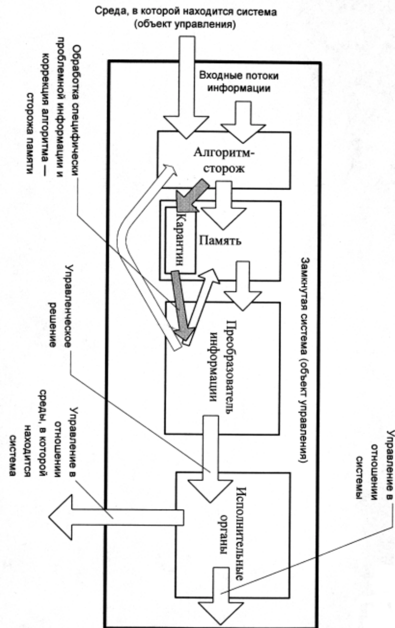
Рис. 3 Алгоритм управления с защитой памяти системы от накопления недостоверной информации
